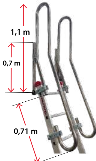
Para pionowych poręczy. Pair of vertical landing handrails.
