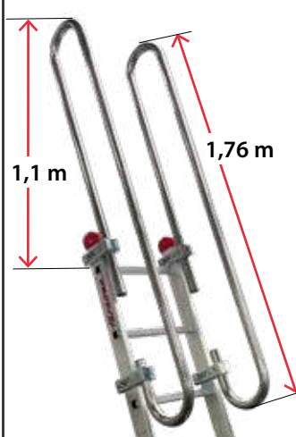
Para pionowych poręczy. Pair of landing handrails.
