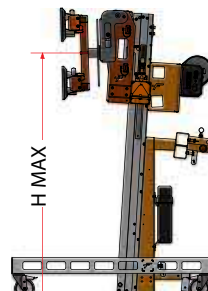
STABILIZACJA PRZEDNIA STD / FRONT STABILIZATION STD
