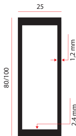
R* - Profil wzmacniony Reinforced profile
