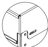
SZCZEGÓŁ B
