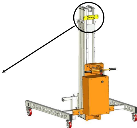
Przykład olinowania
